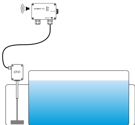
Exemple : Contacteur CF31
